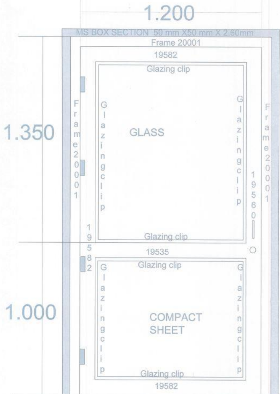
TYP. DETAILS OF DOOR
