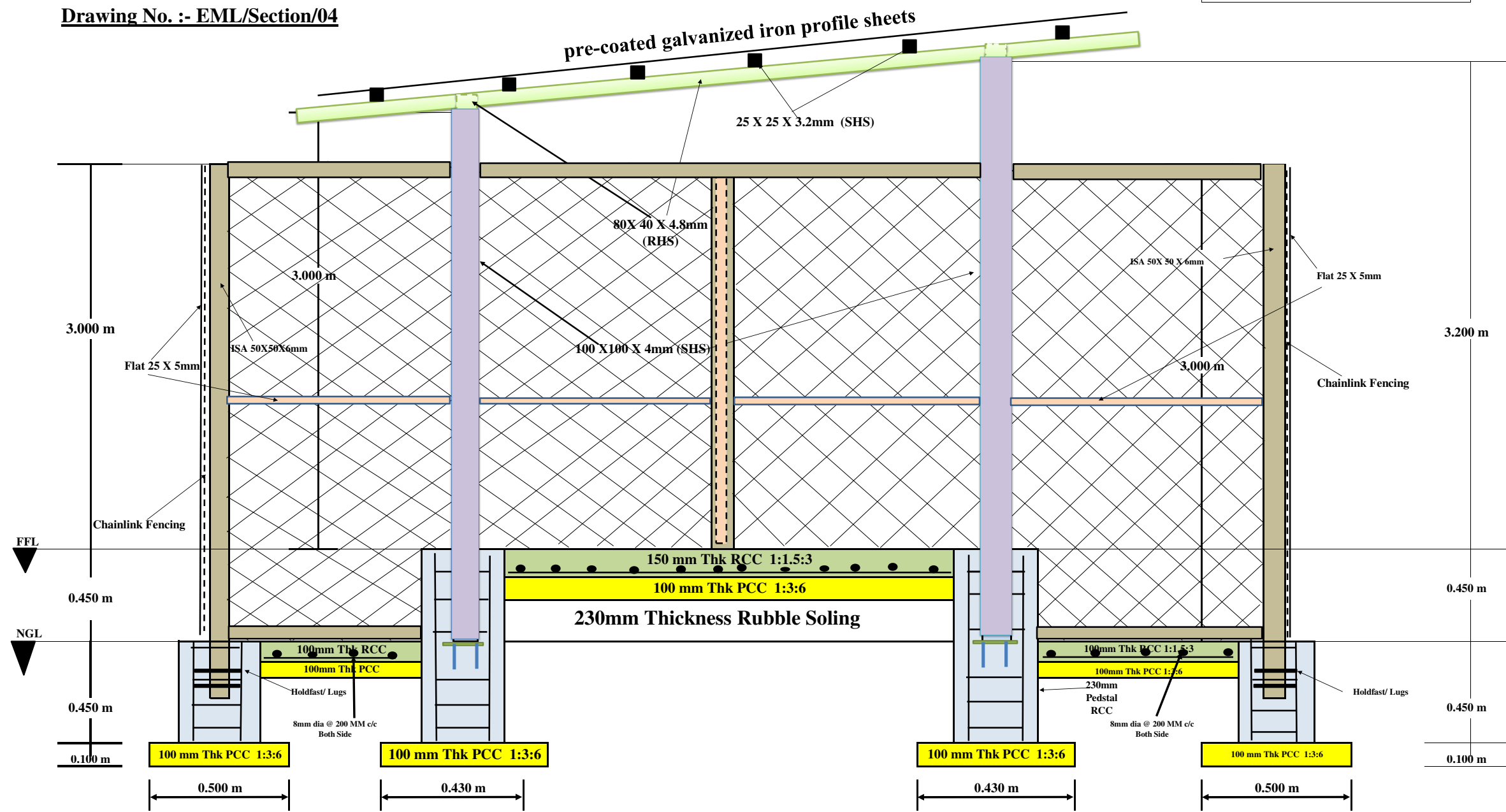
Section D-D
